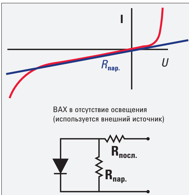
Рис. 2. Вольт-амперная характеристика и эквивалентная схема для затенённого фотогальванического элемента.
