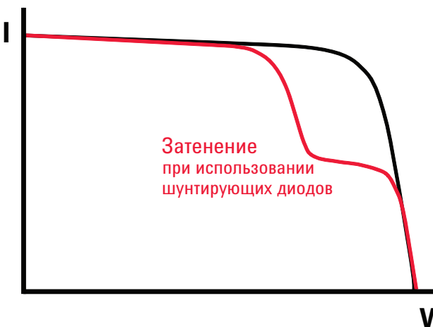
Рис. 11. Некоторые имитаторы солнечных батарей способны воспроизводить работу солнечной батареи в условиях затенения.
