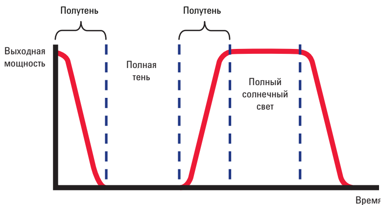
Рис. 8. Выходная мощность изменяется по мере того, как спутник входит, пересекает и покидает область затмения, а затем снова попадает в условия полного солнечного освещения.
