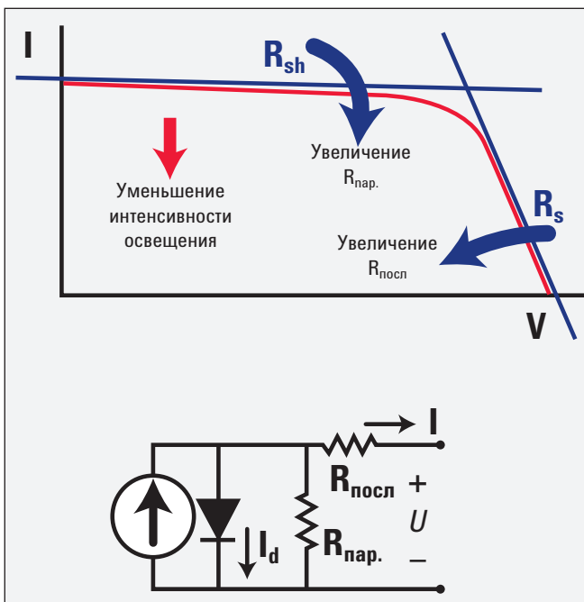
Рис. 1. Вольт-амперная характеристика и эквивалентная схема для облучаемого фотогальванического элемента.
