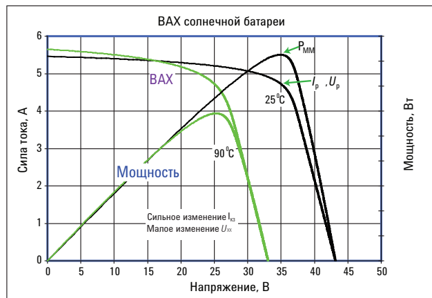
Рис. 5. Перепады температуры оказывают значительное влияние на выходную мощность.
