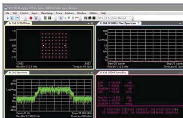
Рисунок 8 - До возникновения помехи: диаграмма созвездия сигнала формата OFDM (слева сверху), модуль вектора ошибки EVM (справа сверху) и спектр (слева внизу) в норме.
